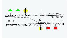
Abb. 10 WVO Bezeichnung von Übergängen: Einfache Bezeichnung eines Übergangs
