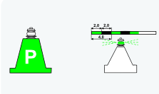
Abb. 4b WVO Tonne mit Licht zur Kennzeichnung von Liegeplätzen auf der linken Seite des Fahrwassers
