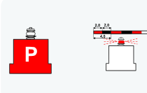
Abb. 4a WVO Tonne mit Licht zur Kennzeichnung von Liegeplätzen auf der rechten Seite des Fahrwassers
