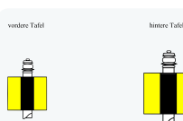
Abb. 11a WVO Bezeichnung der Achse eines langen Übergangs – Zeichenfolge am rechten Ufer (Tafeln)
