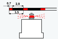
Abb. 1a WVO Rechte Seite des Fahrwassers – Feuer: rotes Taktfeuer
